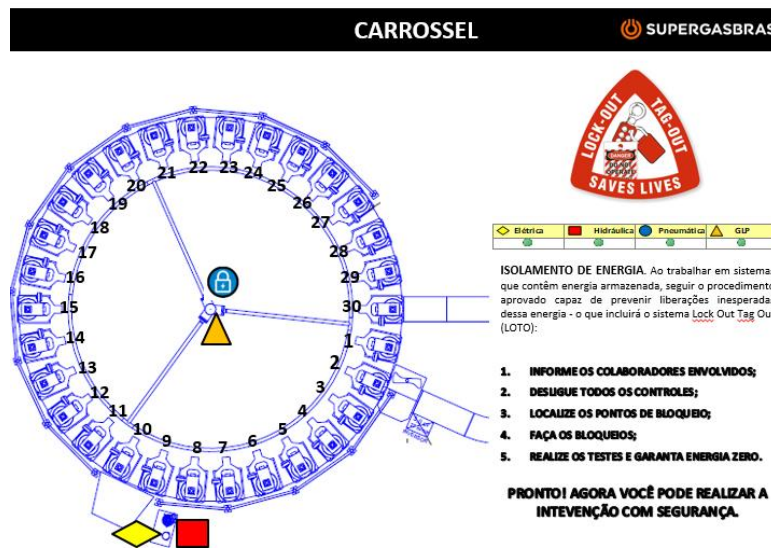
Figura 2 - Modelo LOTO visual
